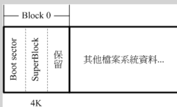
图 6.1.2、4K block 的 boot sector 示意图
